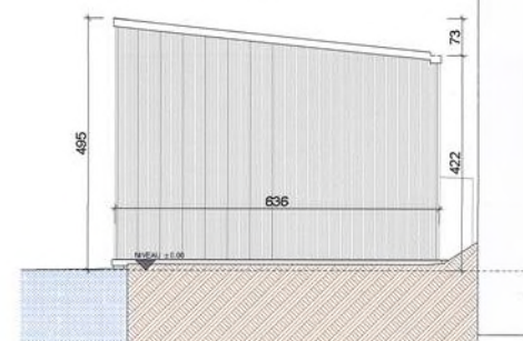
Façade Nord
