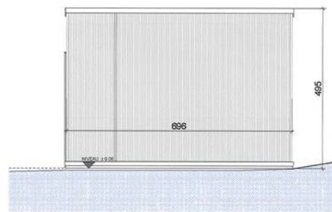
Façade Nord
