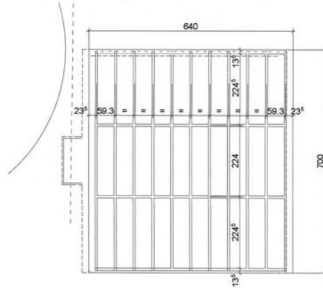
Charpente métallique
