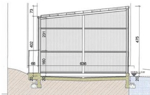
Coupe B-B
