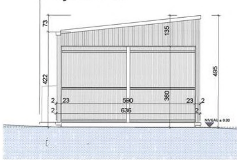
Façade Sud
