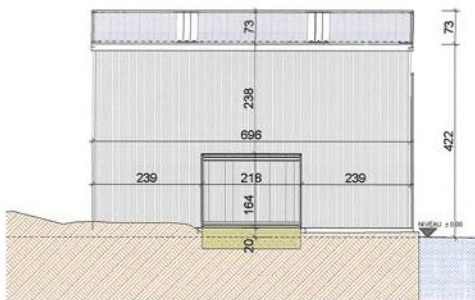
Coupe B-B
