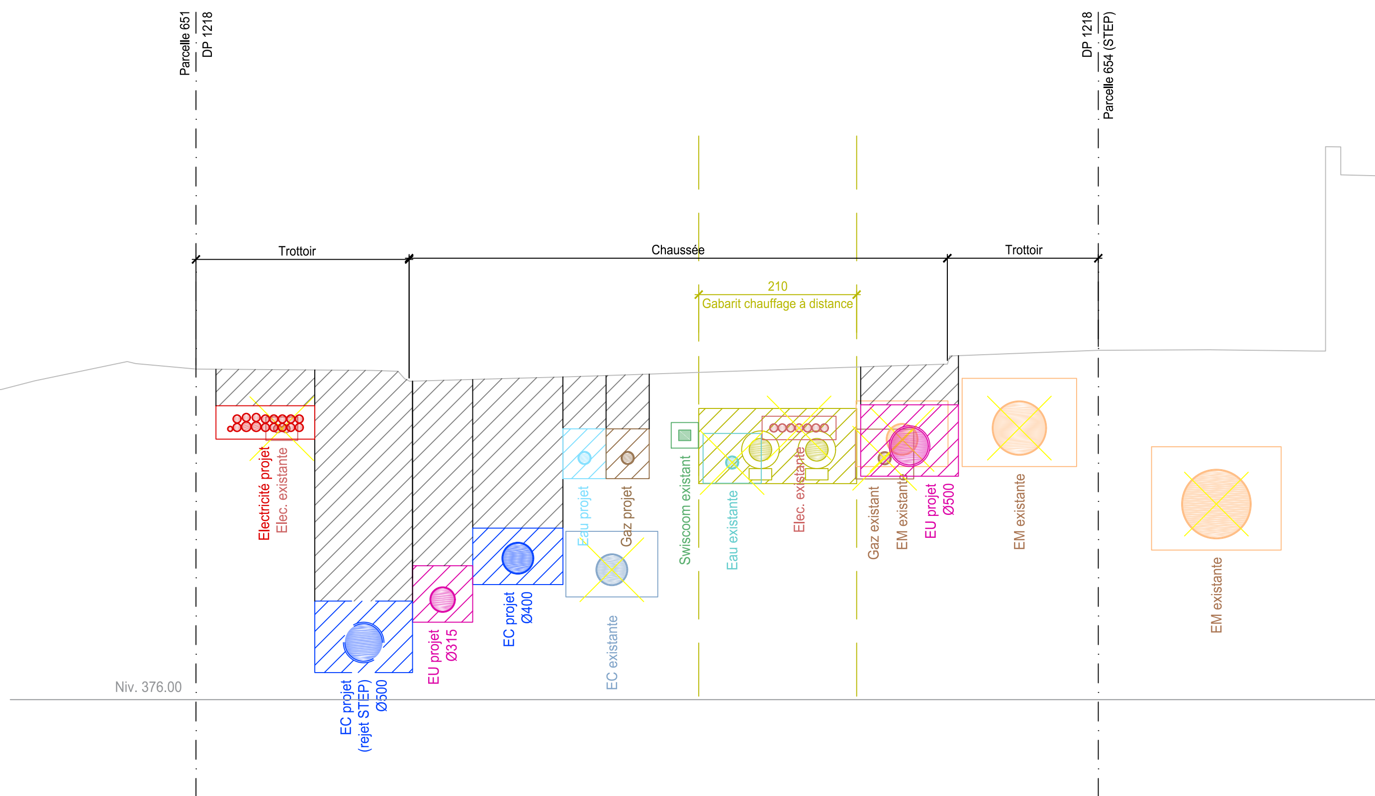
PROFIL EN TRAVERS N°22 1:50
