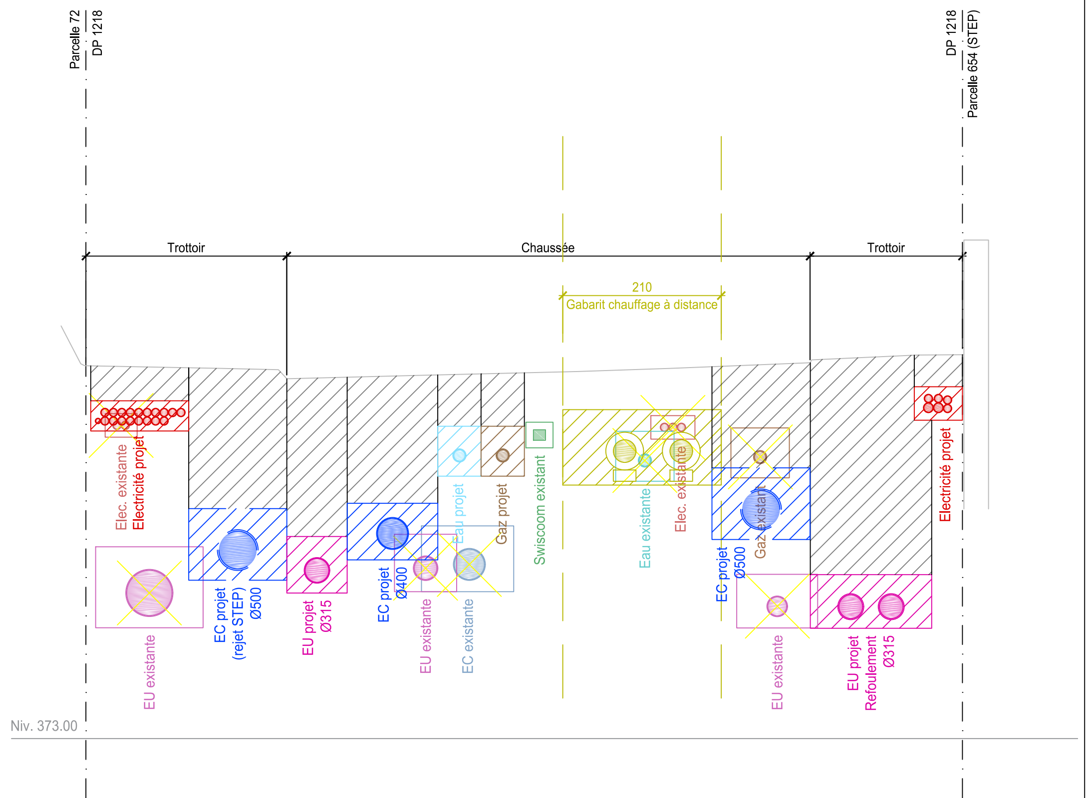
PROFIL EN TRAVERS N°12 1:50
