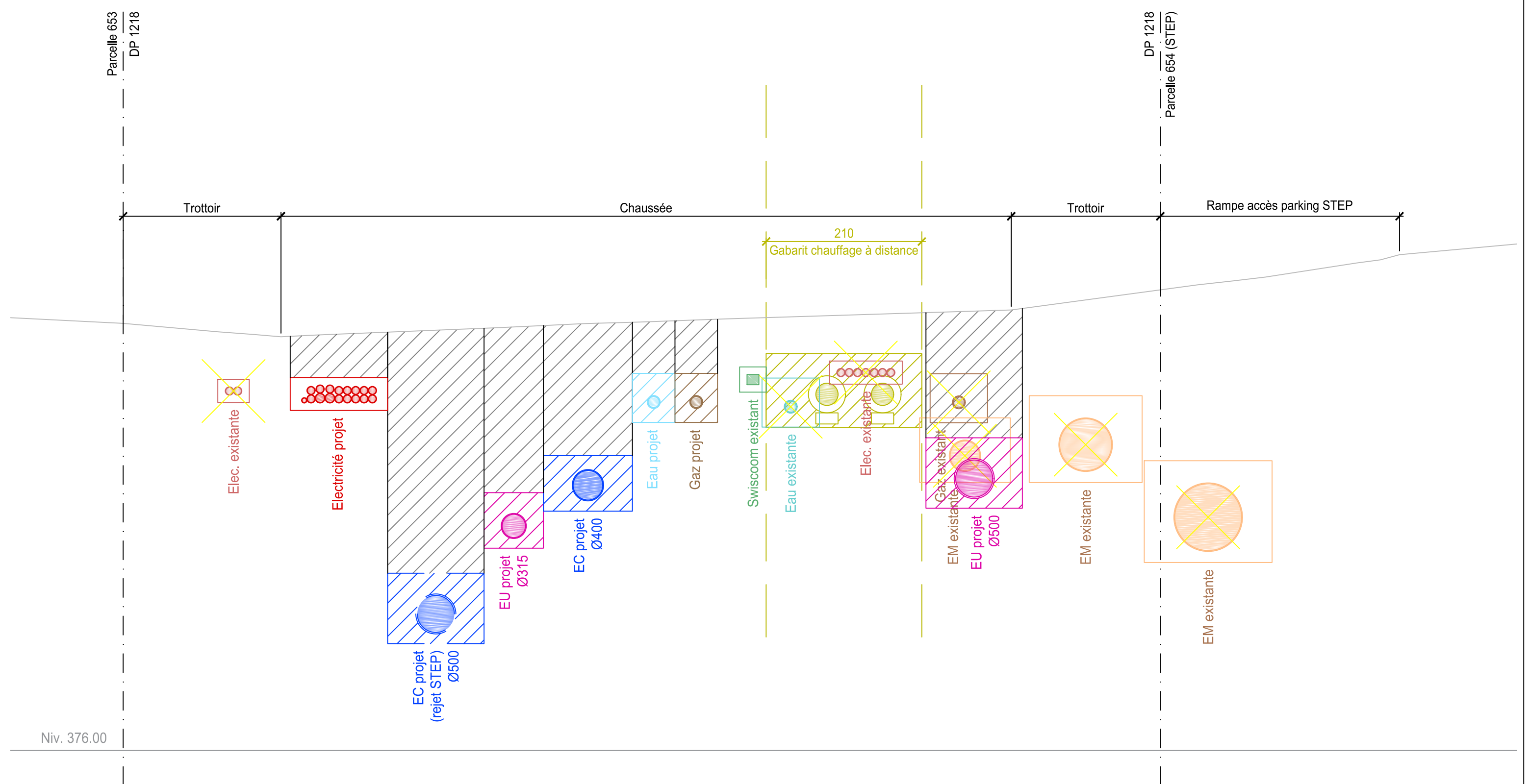
PROFIL EN TRAVERS N°27 1:50
