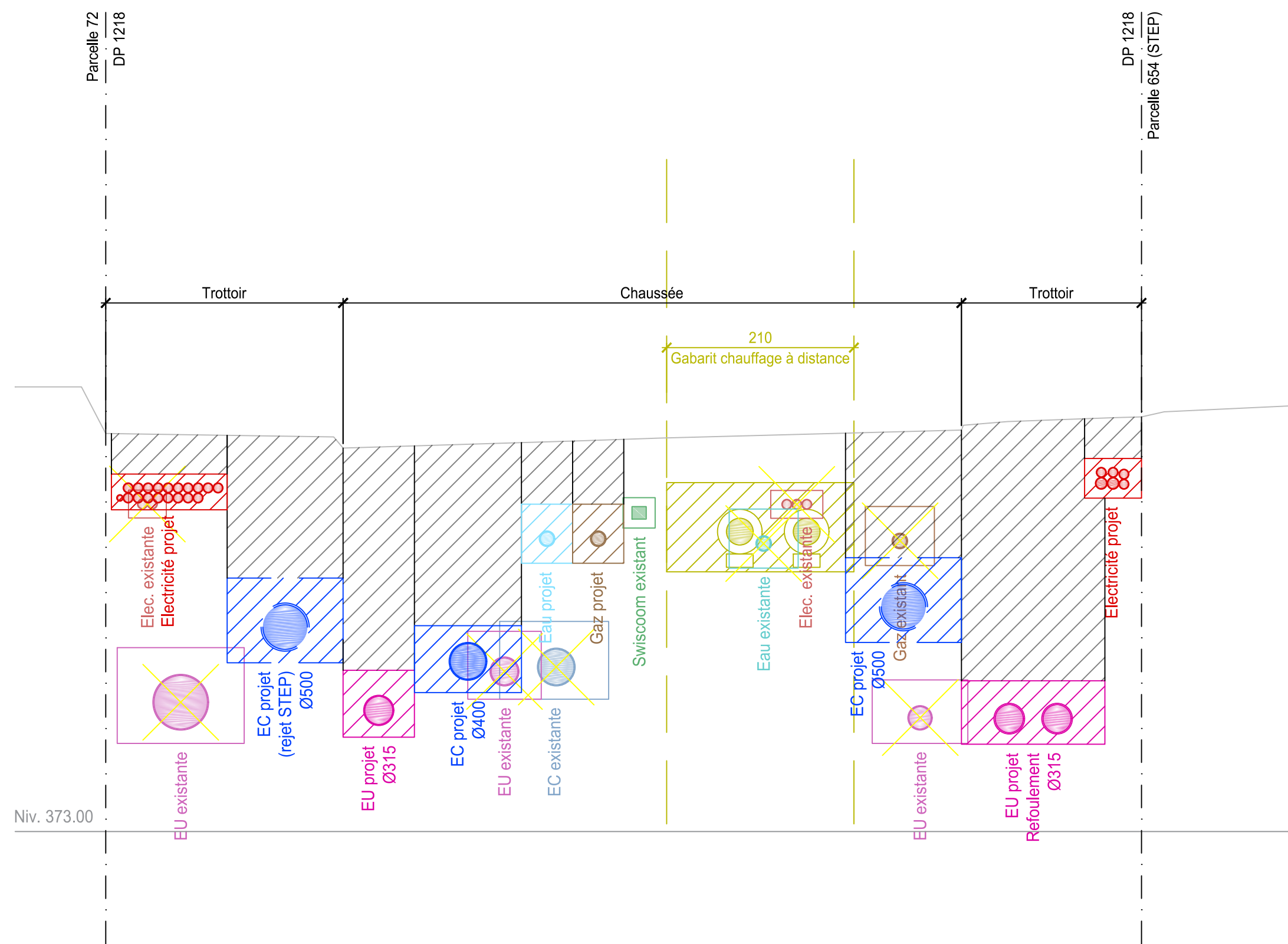
PROFIL EN TRAVERS N°11 1:50
