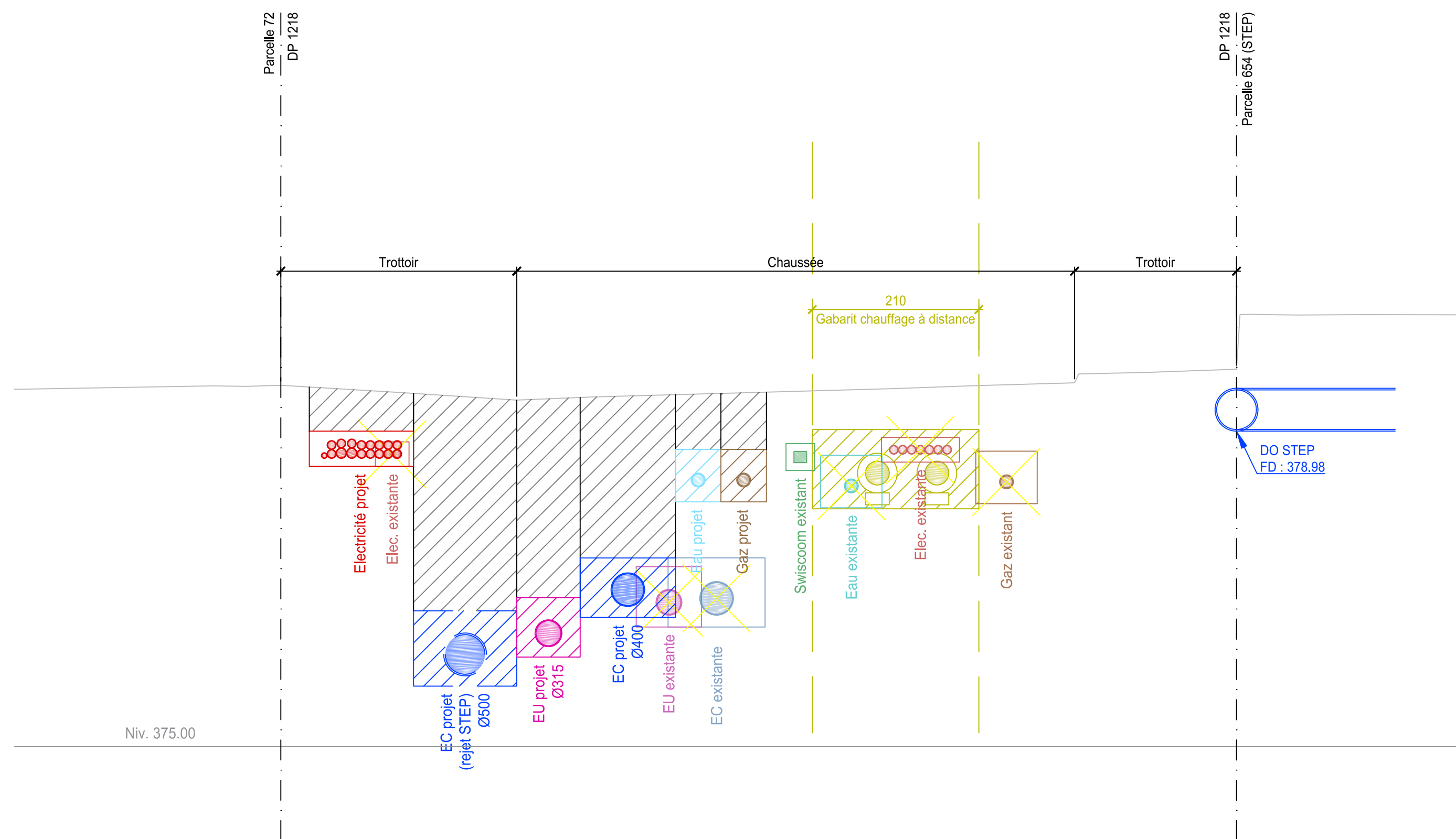
PROFIL EN TRAVERS N°16 1:50
