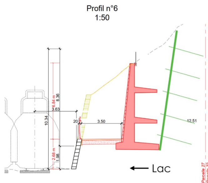
Figure 6 : coupe du chemin de mobilité active pour accéder à la passerelle du côté de Belmont-sur-Lausanne. © Gruner.
