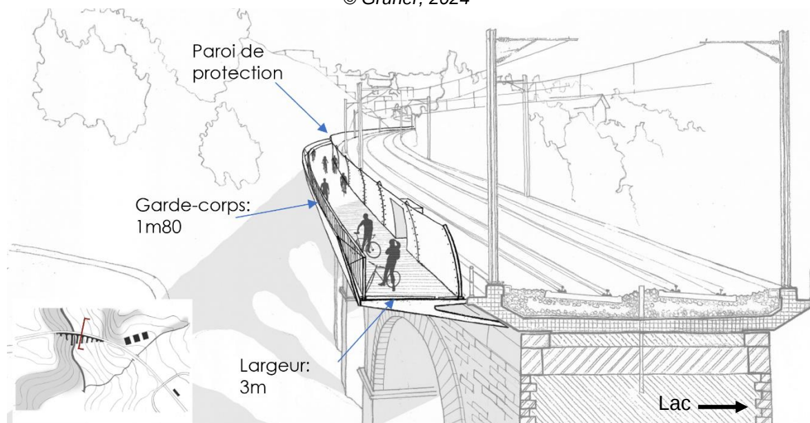
Figure 3 : coupe de la passerelle le long du viaduc CFF de Rochettaz. © Glatz & Delachaux, 2024
