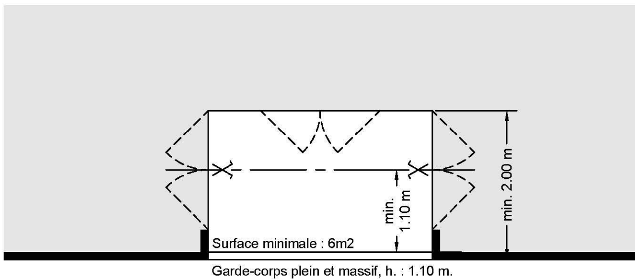
Figure 1, Article 27, alinéas 5 et 6, loggia ou balcon fermés,
