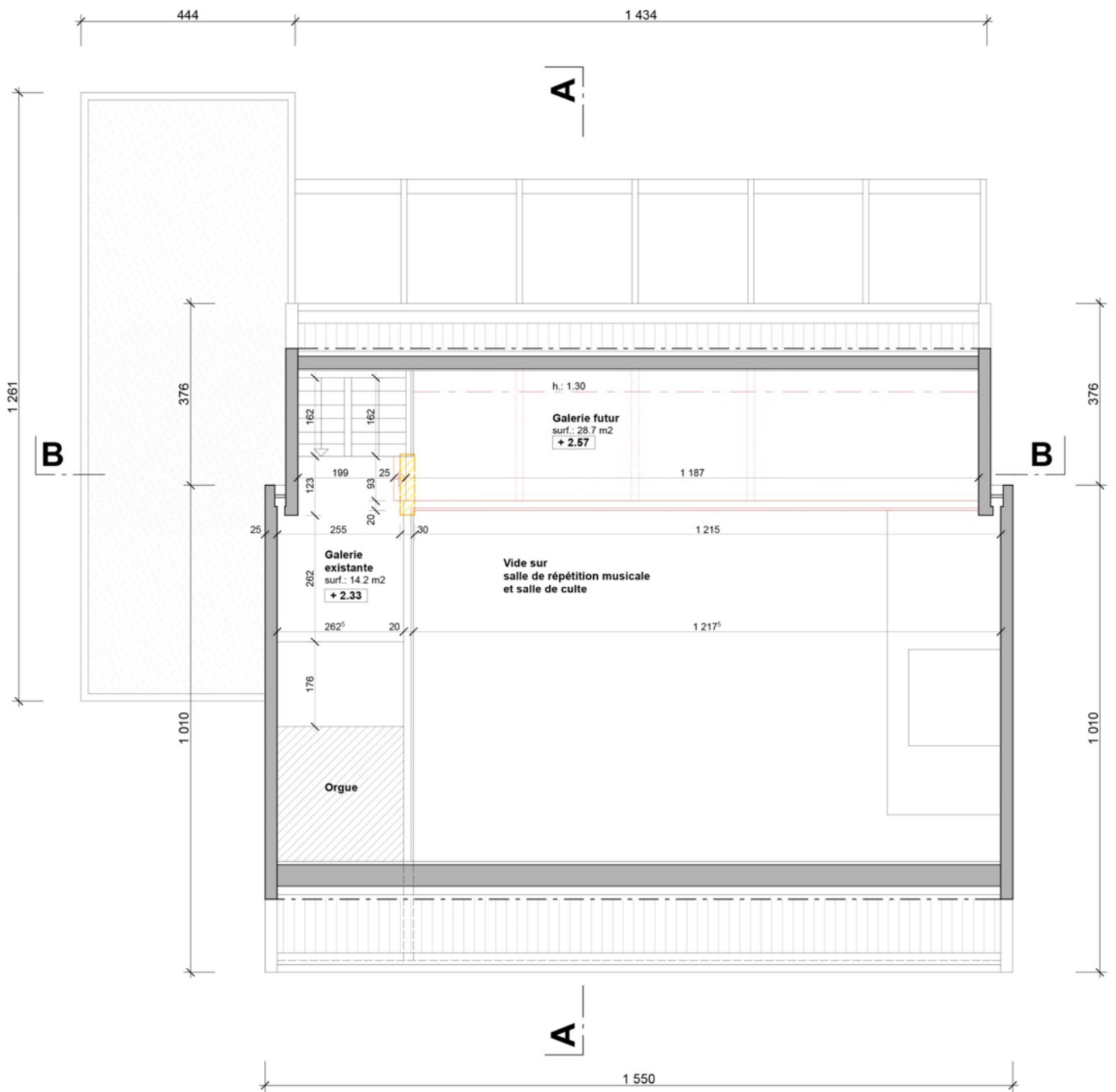
Galerie état futur
