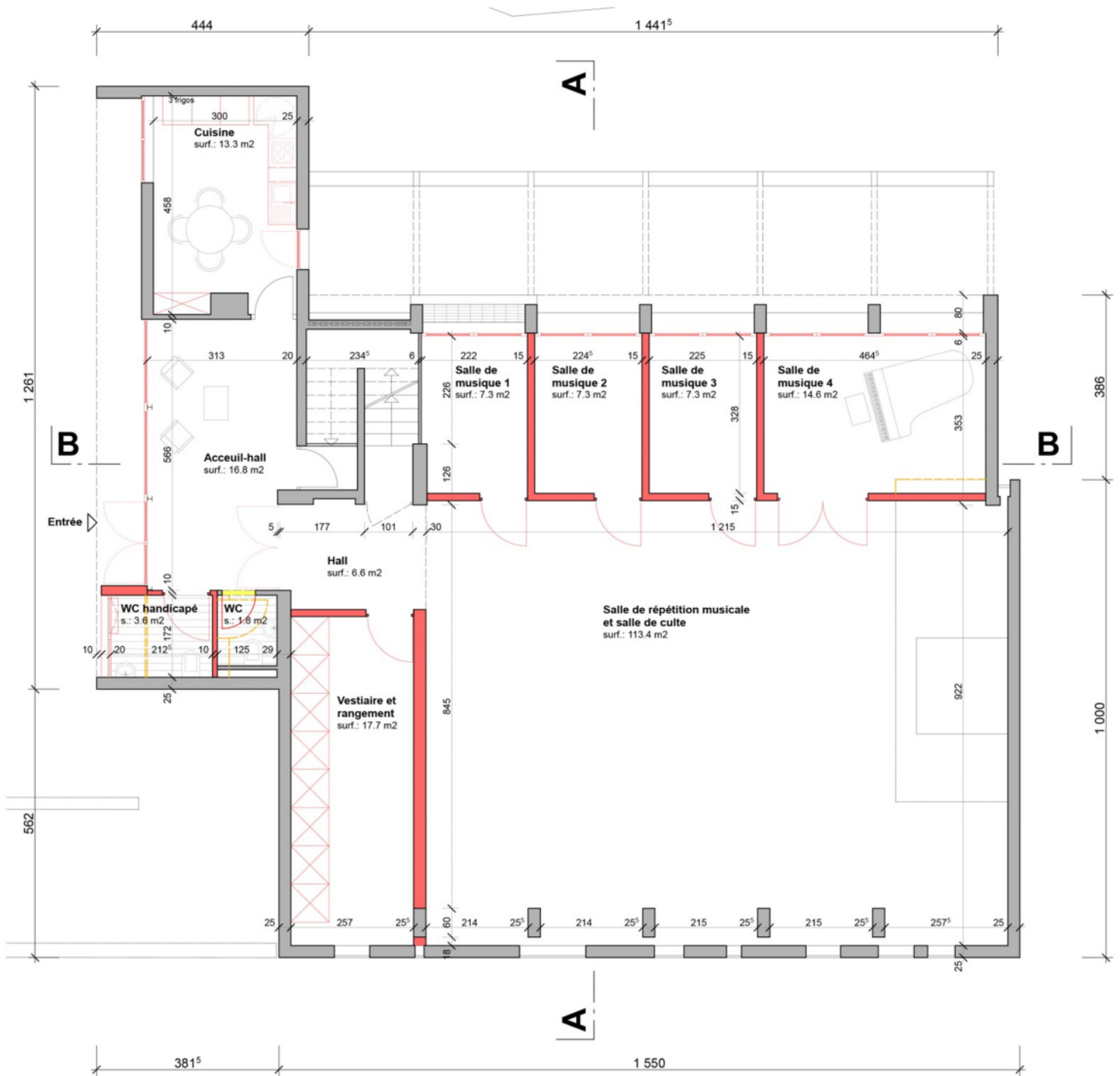
Rez supérieur état futur
