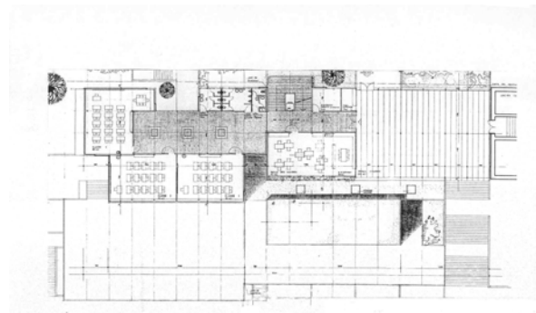
Niveau 000
