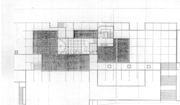
Niveau + 1020
