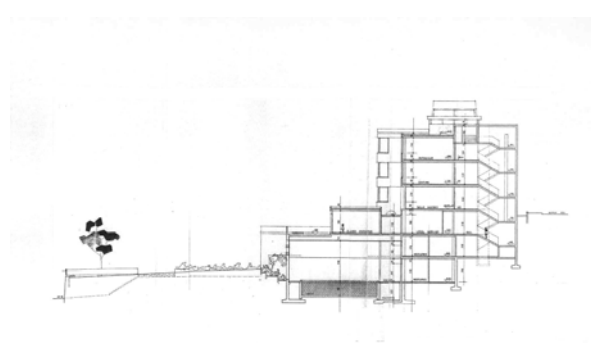
Coupe
