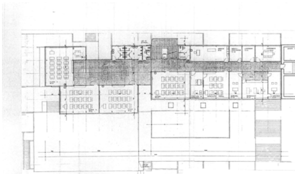
Niveau + 340
