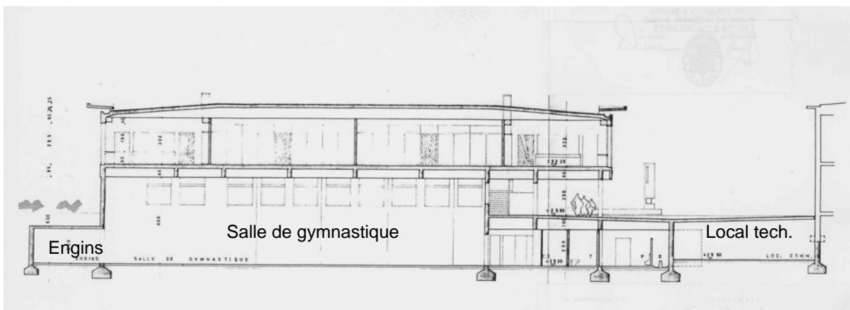
COUPE LONGITUDINALE
