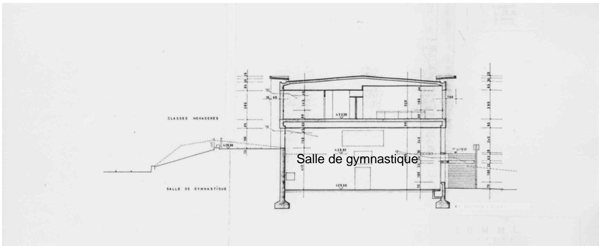
COUPE TRANSVERSALE
