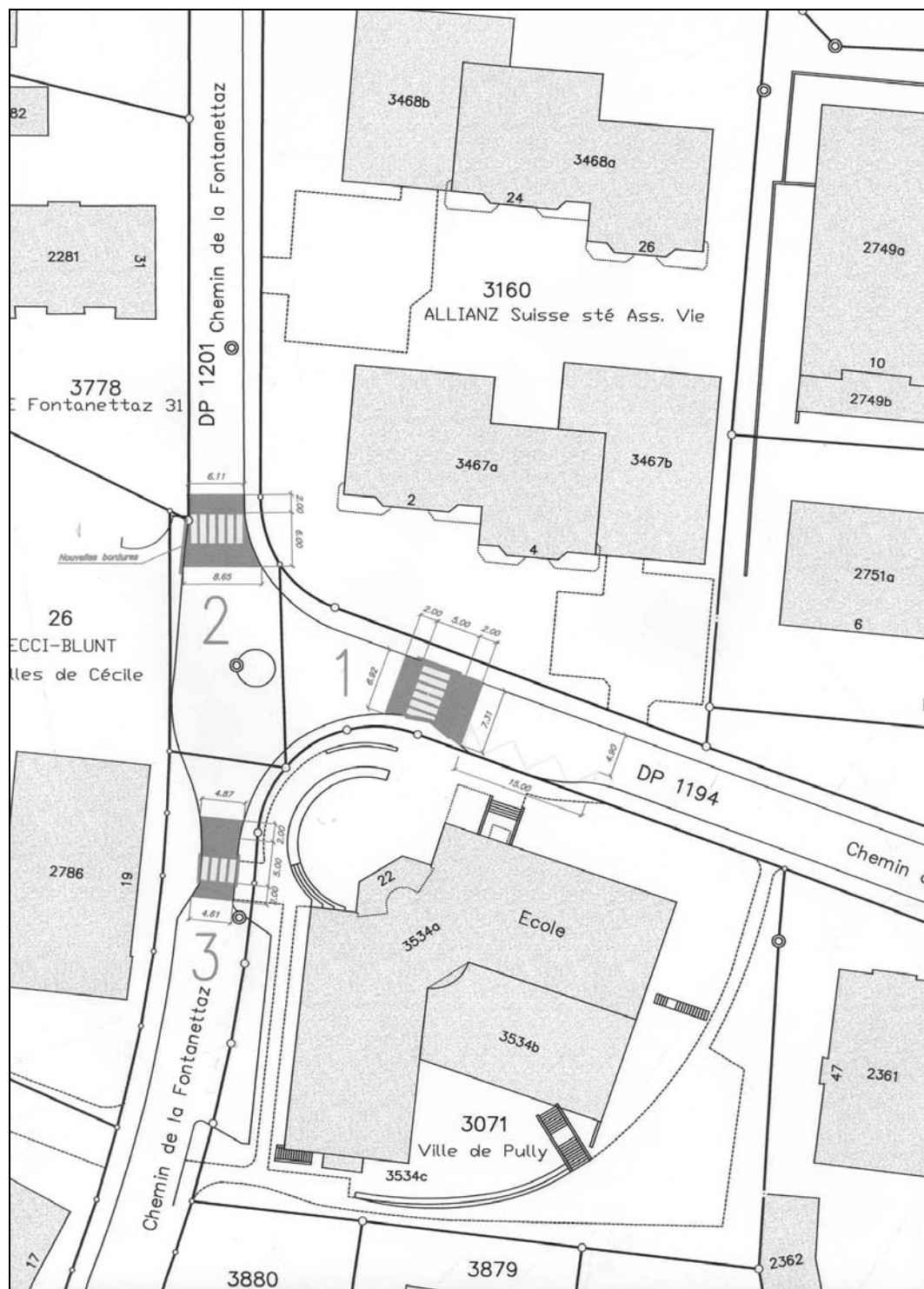
Projet des trois seuils ralentisseurs
