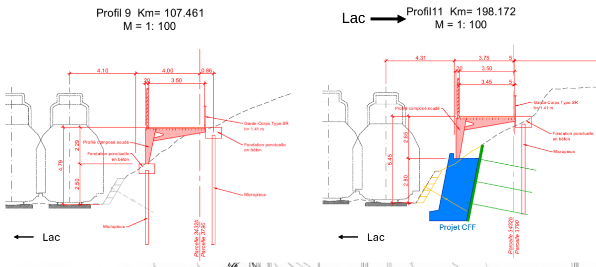
Figure 4 : coupes du chemin de mobilité active pour accéder à la passerelle du côté de Pully
