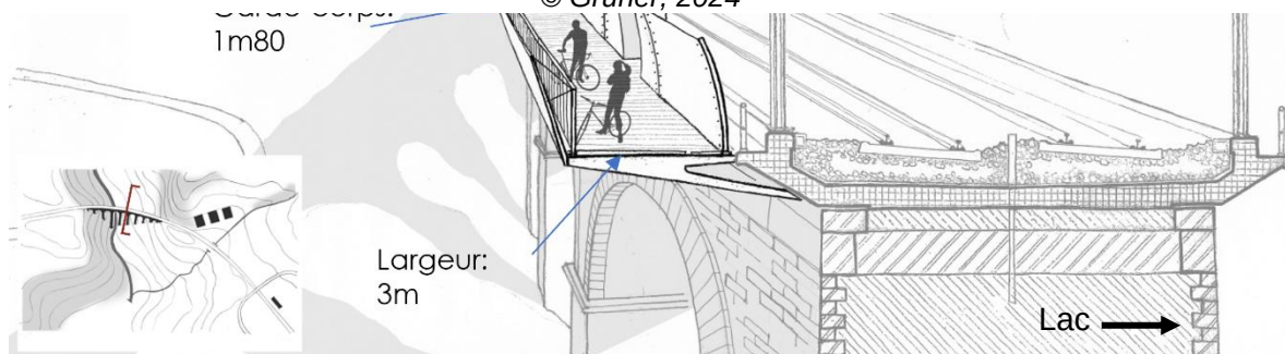
Figure 3 : coupe de la passerelle le long du viaduc CFF de Rochettaz. © Glatz & Delachaux, 2024
